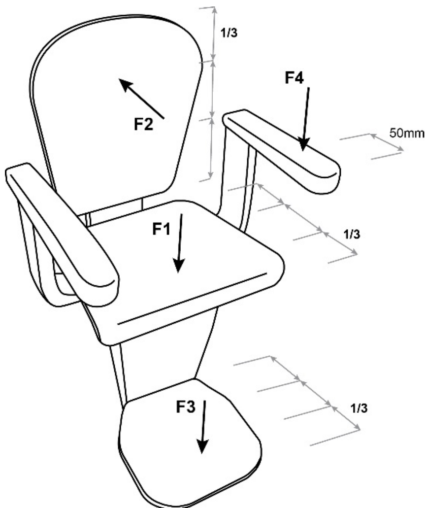
Рисунок Б.1 – Схема приложения нагрузки. Ремень безопасности испытывается отдельно от кресла
