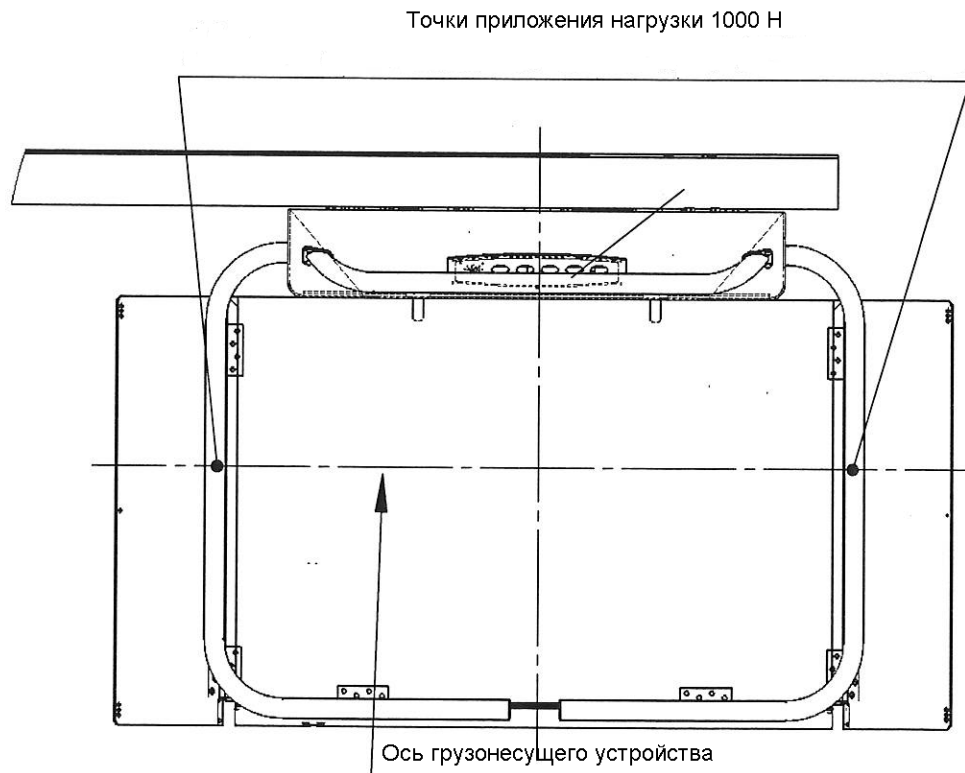
Рисунок Б.4 — Точки приложения нагрузки 1000 Н
